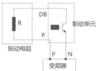
典型电路图
